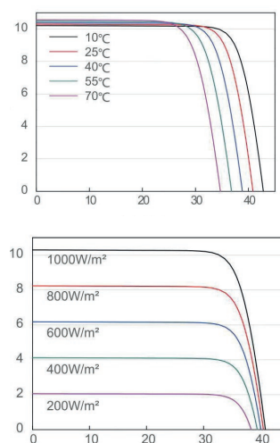
Wykres prąd-napięcie: (A-HCM320M)
